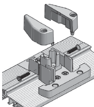
Łącznik słupka stałego (MH...) tworzywowy z wiatrostopem i uszczelką samoprzylepną
